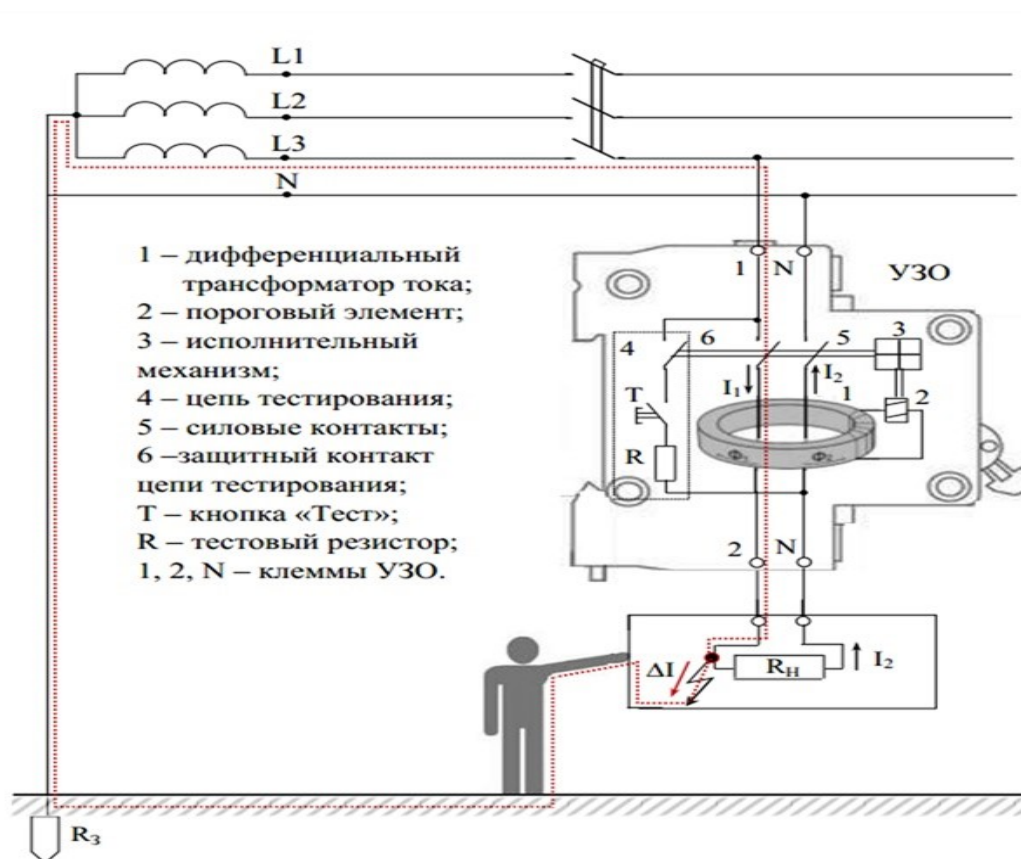
Рисунок 3. Принцип работы УДТ
